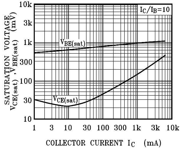
V_{CE(sat)}, V_{BE(sat)} - I_C
